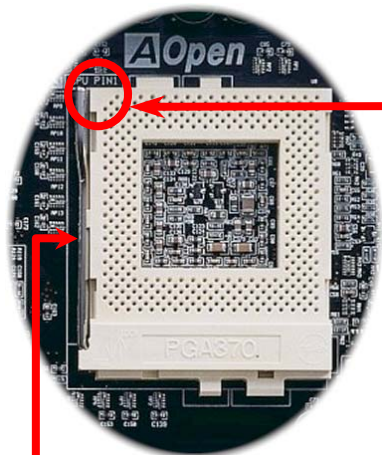
CPU 插座固定桿
