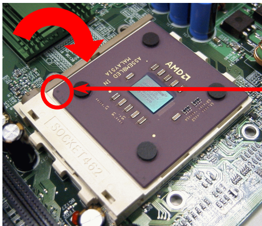
CPU 缺角記號
