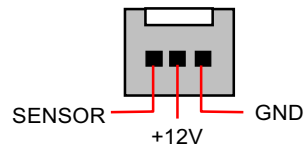
CPU ファンコネクタ
