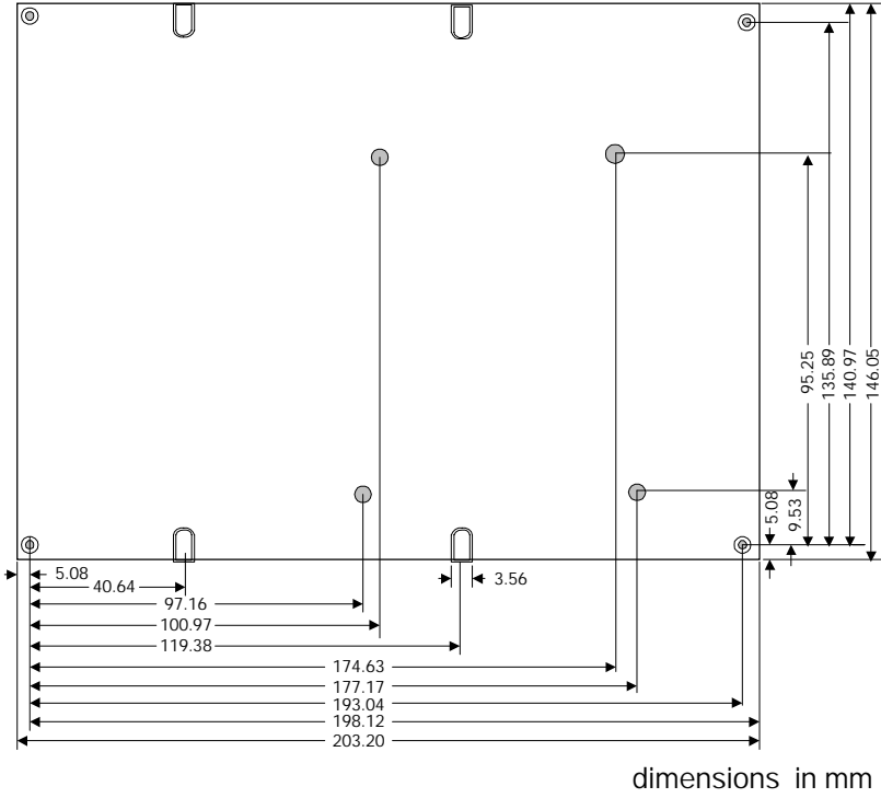
PCM-7890 dimensions
