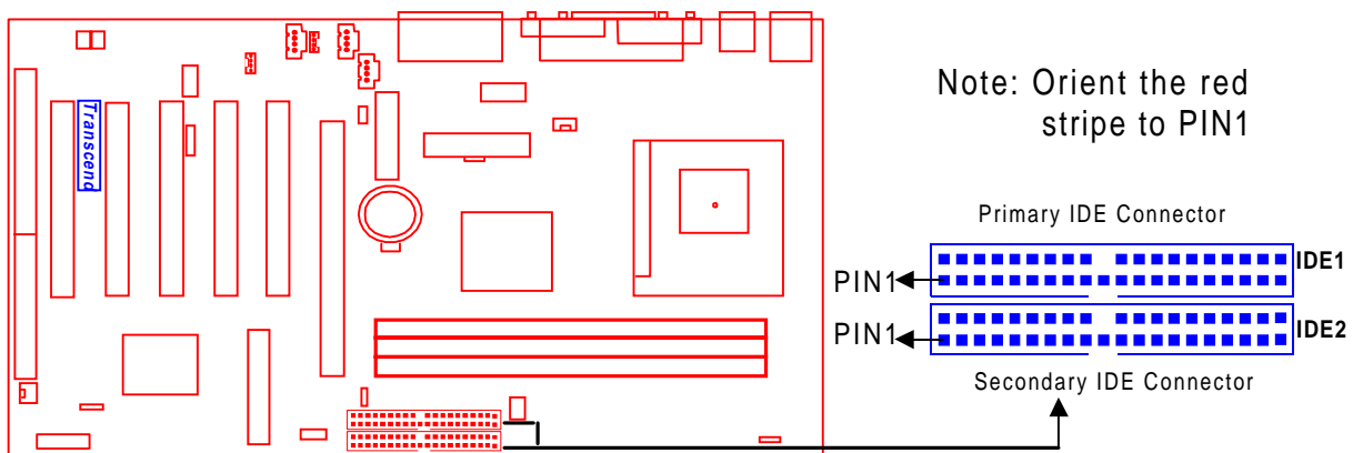
IDE Connectors
