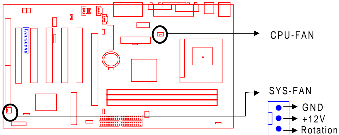
Fan Power Connectors
