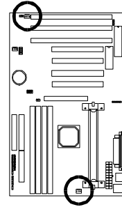
CPU Fan Connector
