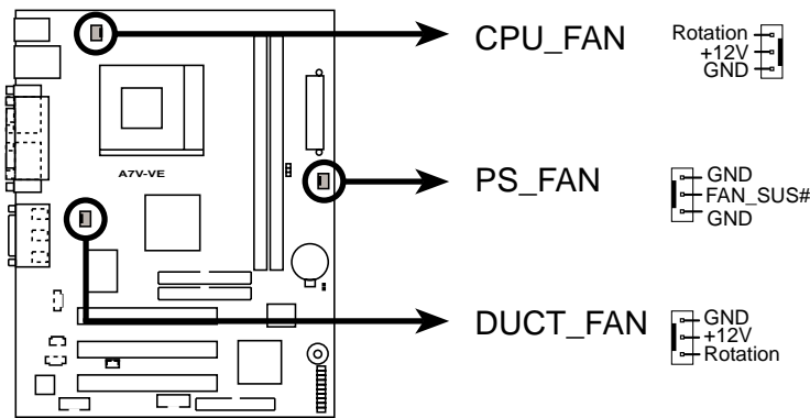
A7V-VE 12-Volt Cooling Fan Power
