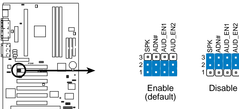
P3W Audio Codec Setting
